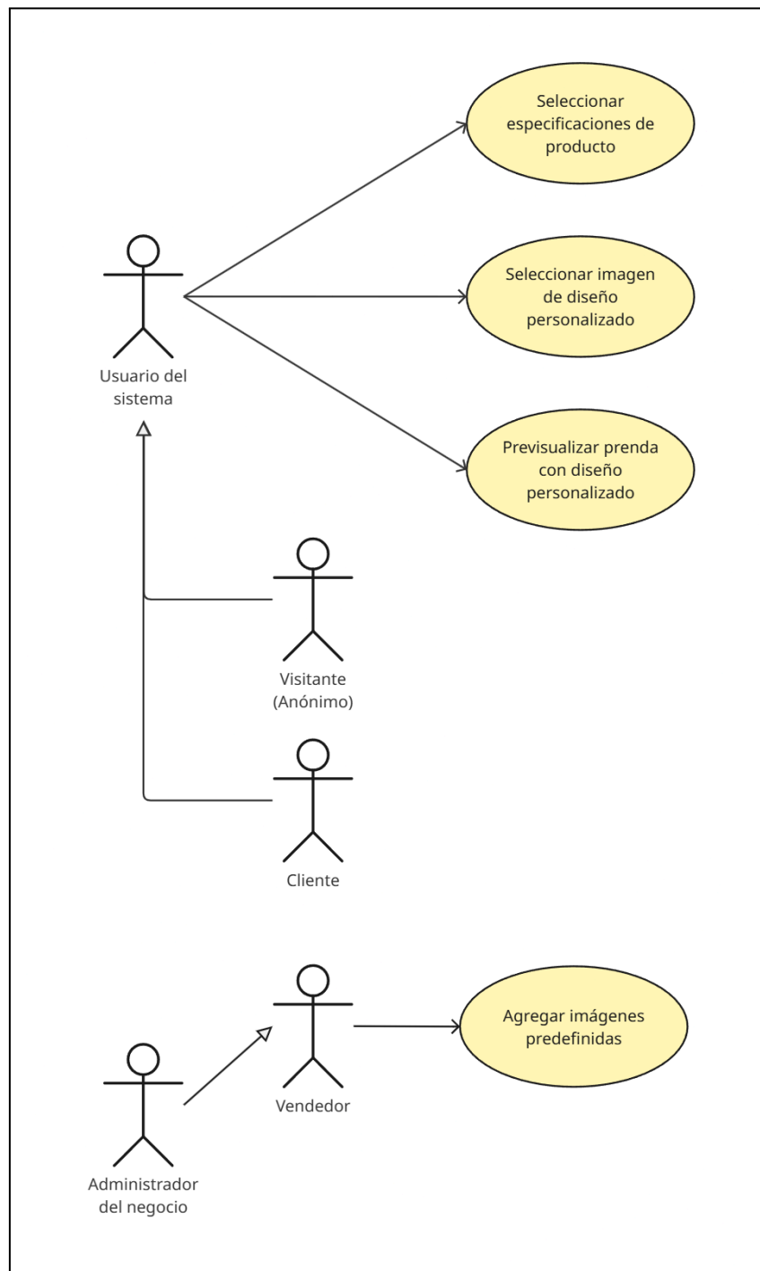
Figura 4: Diagrama de Casos de Uso de Personalización de Productos
