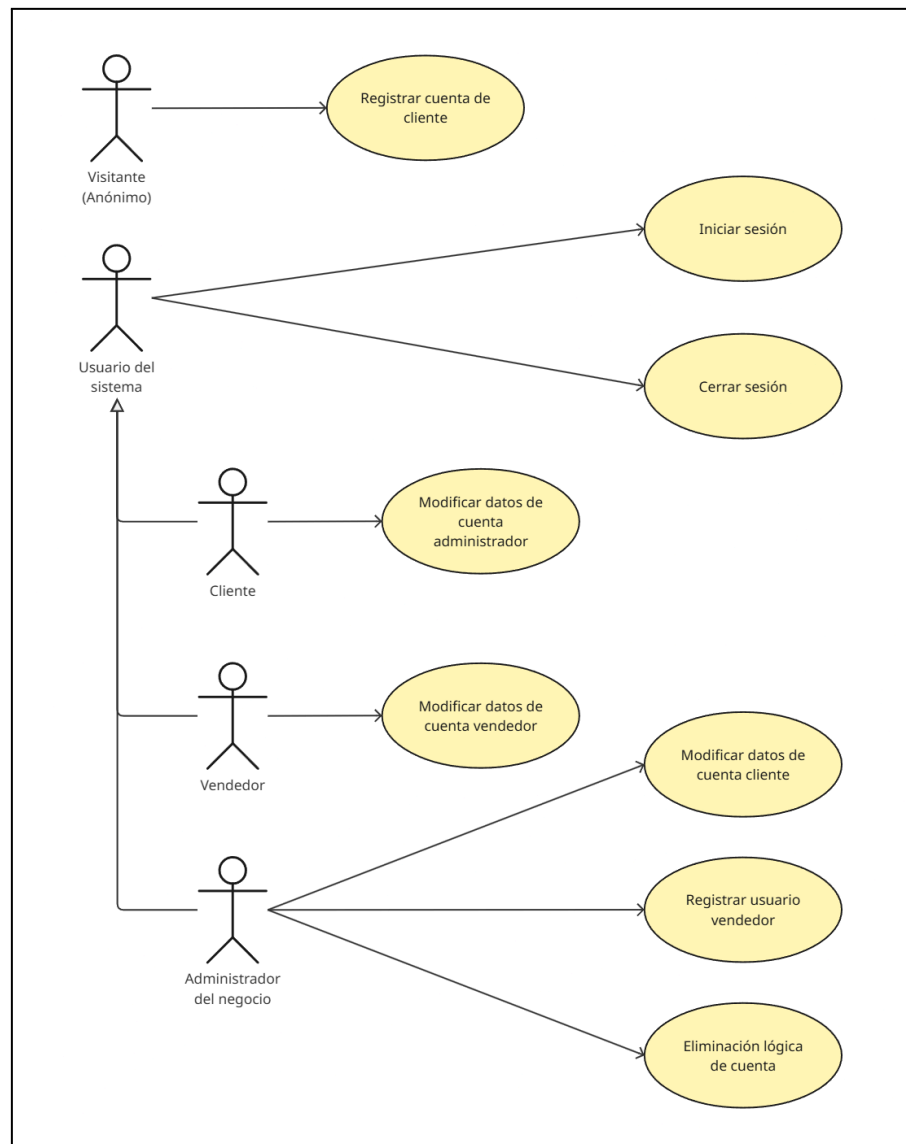
Figura 2: Diagrama de Casos de Uso de Gestión de Acceso y Usuarios
