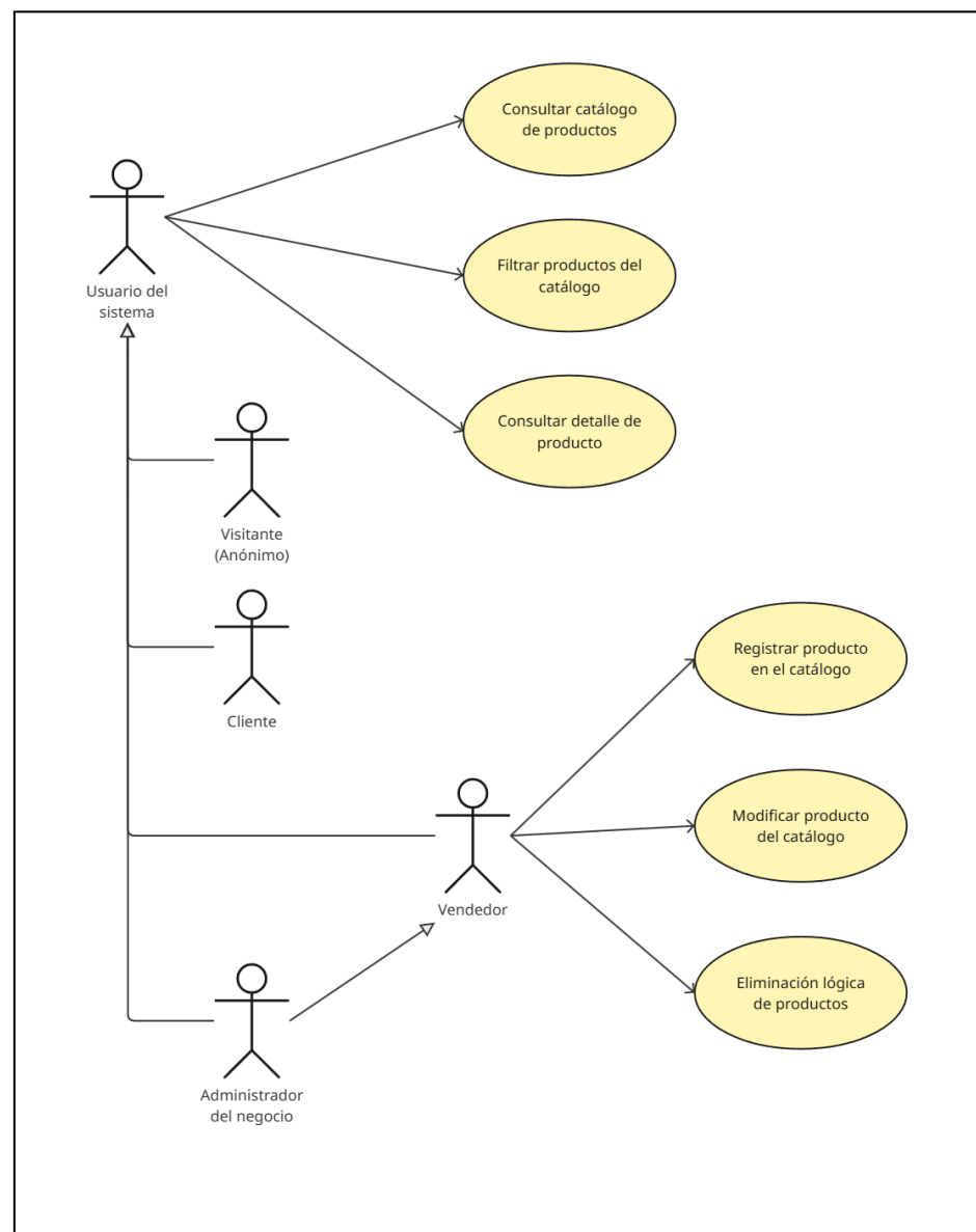
Figura 3: Diagrama de Casos de Uso de Manejo y Gestión del Catálogo de Productos
