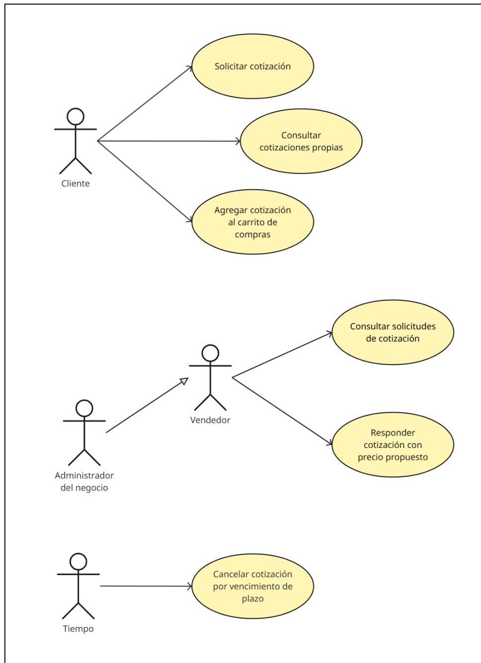
Figura 6: Diagrama de Casos de Uso de Cotizaciones de Pedidos
