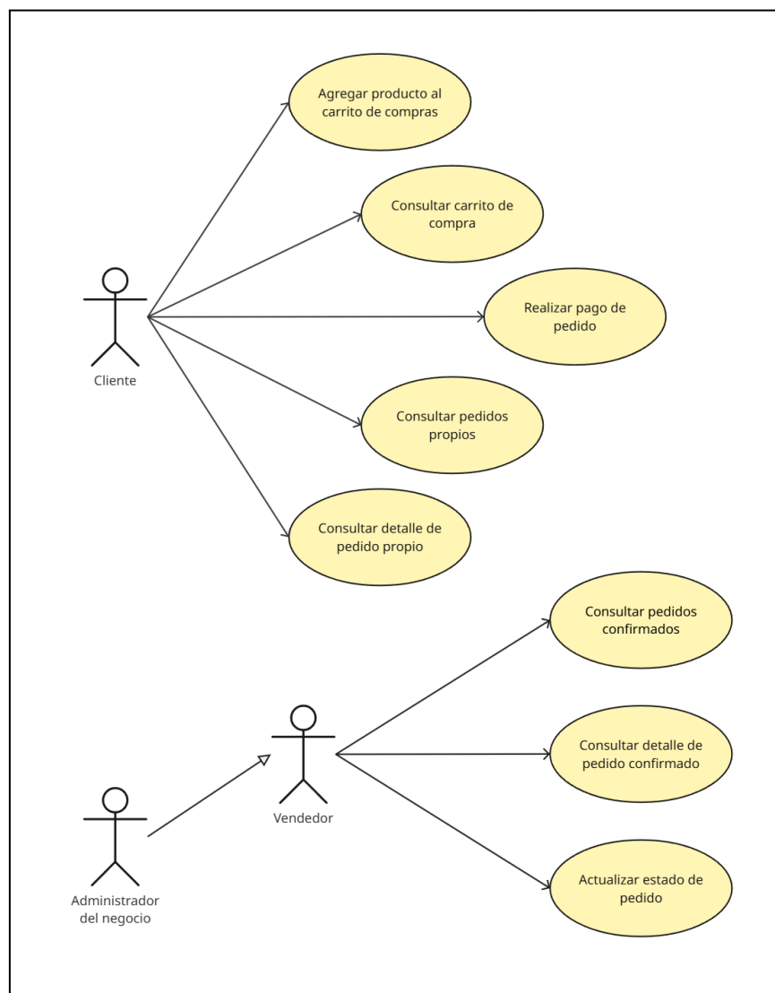
Figura 5: Diagrama de Casos de Uso de Gestión de Ventas y Pedidos
